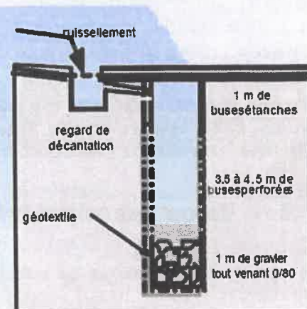
PUITS D'INFILTRATION D'EAUX DE PLATEFORME ROUTIERE
