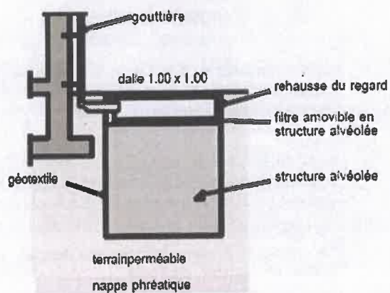
PUITS D'INFILTRATION INDIVIDUEL
